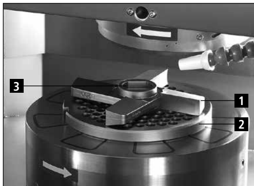
Figure 7-16 Couteaux sur table circulaire
