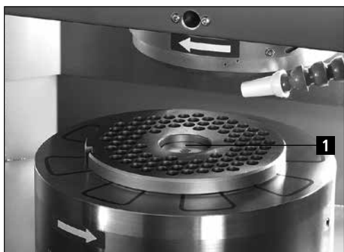
Figure 7-15 Disque d'affûtage sur table circulaire
