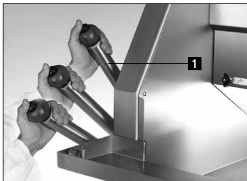
Figure 7-4 Levier de commande «Table circulaire»
