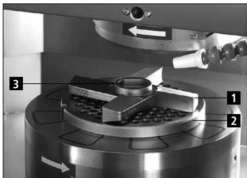
Figure 7-11 Couteaux sur table circulaire
