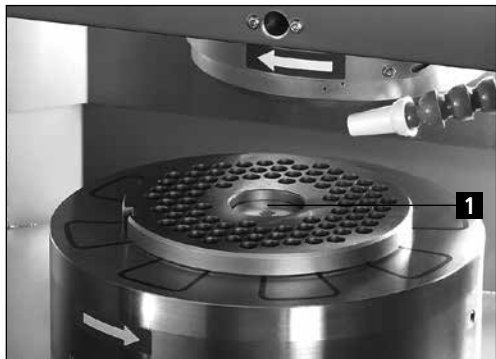
Figure 7-8 Disque d'affûtage sur table circulaire
