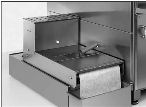
Figure 6-1 Remplir l'installation de liquide de refroidissement à bande filtrante
