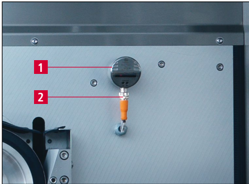
Bild 9-7 Strömungswächter
