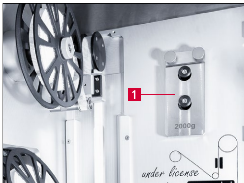
Bild 7-23 Kalibriergewicht abnehmen
