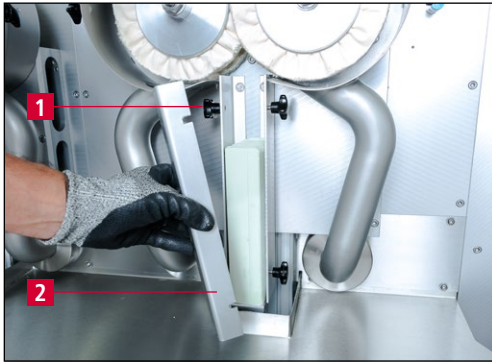
Bild 7-16 Polierpaste wechseln
