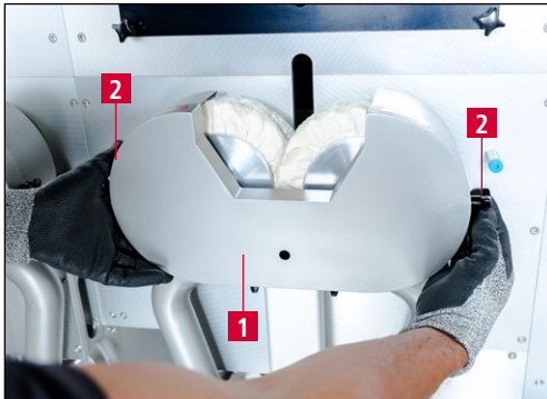
Bild 7-14 Schutzhaube abnehmen
