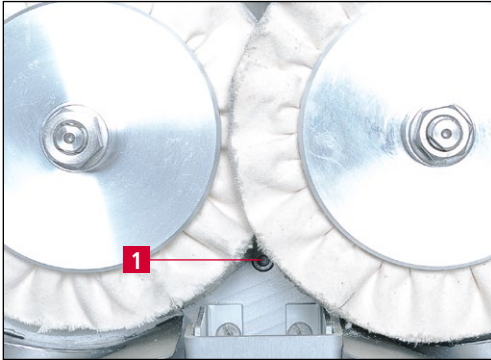
Bild 7-17 Polier-/Entgratringe einstellen
