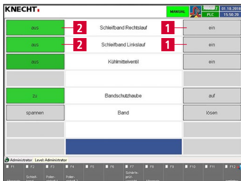
Bild 7-12 Handfunktionen „Schleifband“
