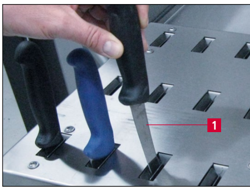
Bild 7-1 Messermagazin
