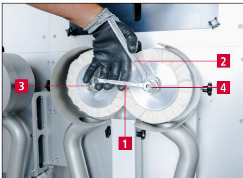
Bild 7-15 Polier-/Entgratringe wechseln
