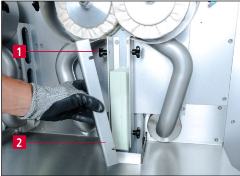
Bild 7-16 Polierpaste wechseln
