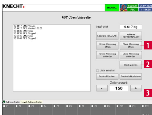
Bild 7-28 Einstellungen Schärfprüfvorrichtung
