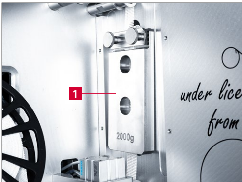
Bild 7-25 Kalibriergewicht
