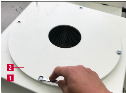
Bild 9-5 Filterdeckel
