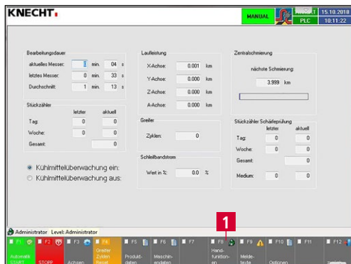
Bild 7-10 Einstellungen
