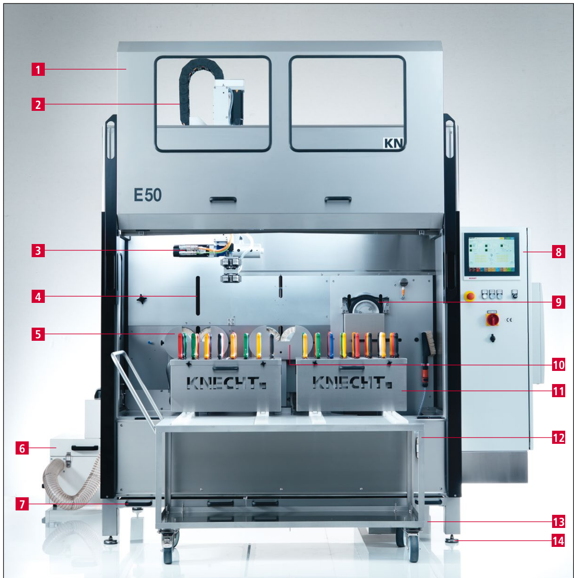
Bild 3-2 Gesamtansicht Schleifmaschine
