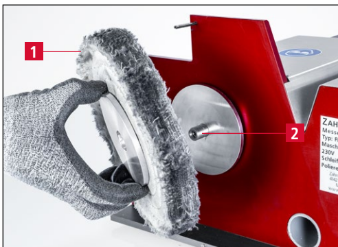
Bild 7-14 Spannflansch und Polierscheibe abnehmen
