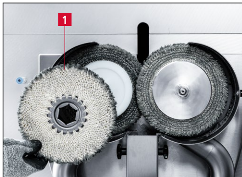
Bild 7-26 Gebrauchten Entgratring abnehmen
