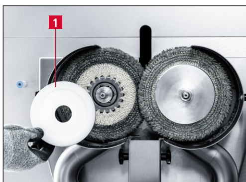
Bild 7-27 Zwischenflansch abnehmen
