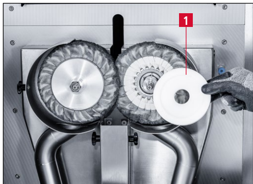
Bild 7-44 Zwischenflansch abnehmen
