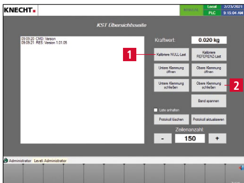
Bild 7-65 „NULL-Last“ kalibrieren
