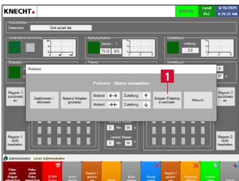
Bild 7-38 Polieren – Polierringe wechseln
