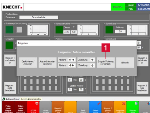
Bild 7-21 Entgraten – Entgratringe wechseln
