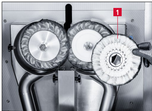
Bild 7-43 Gebrauchten Polierring abnehmen
