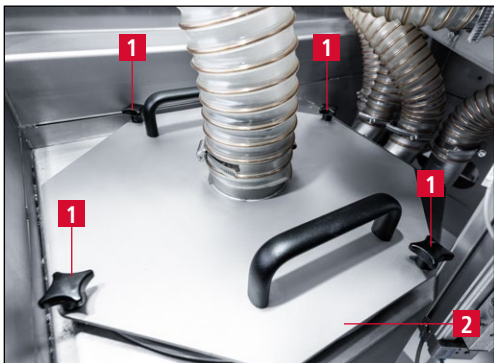
Bild 9-3 Absauganlage öffnen
