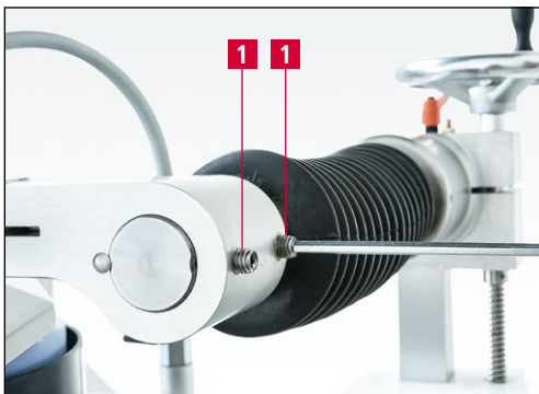
Bild 6-5 Kreismesserschleifeinrichtung festziehen
