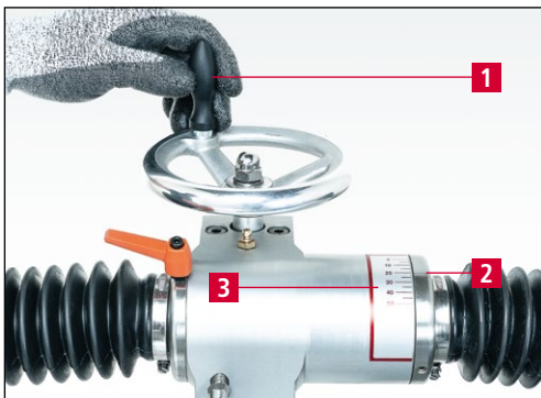
Bild 7-11 Schleifwinkel einstellen
