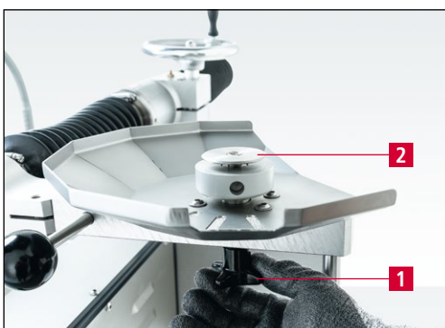
Bild 7-3 Messeraufnahme abnehmen
