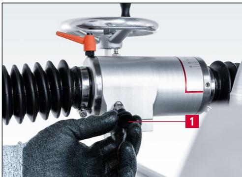
Bild 6-1 Rastbolzen einrasten
