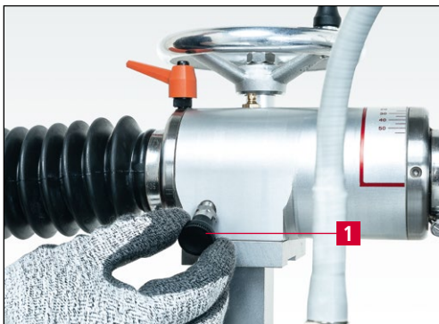
Bild 7-2 Rastbolzen lösen
